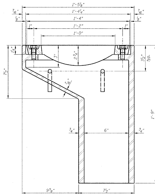
SECTION A-A
