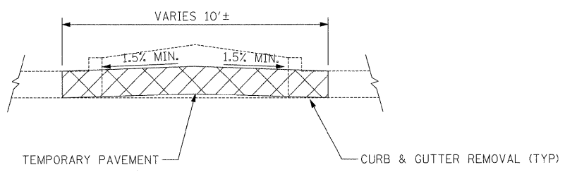
SECTION A-A (STA. 249+00 TO STA. 255+00) (N.T.S.)
