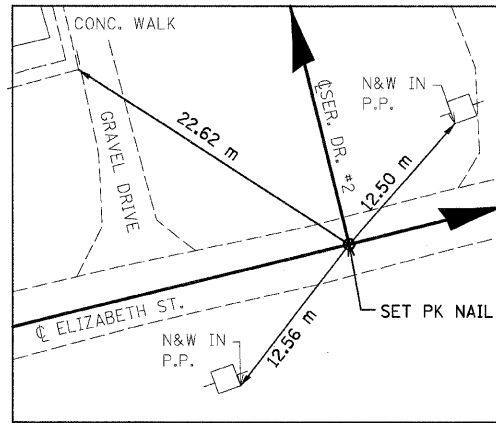
ELIZABETH STREET STA 0+152.000 SERVICE DRIVE 2 STA 0+000.000 N 255,680.1081 E 698,276.7393
