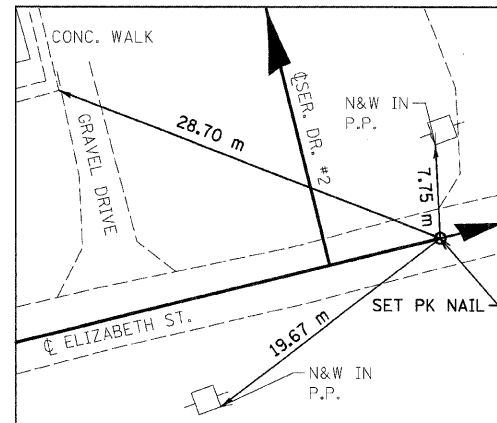
ELIZABETH STREET POT STA 0+160.000 N 255,682.0202 E 698,284.5075
