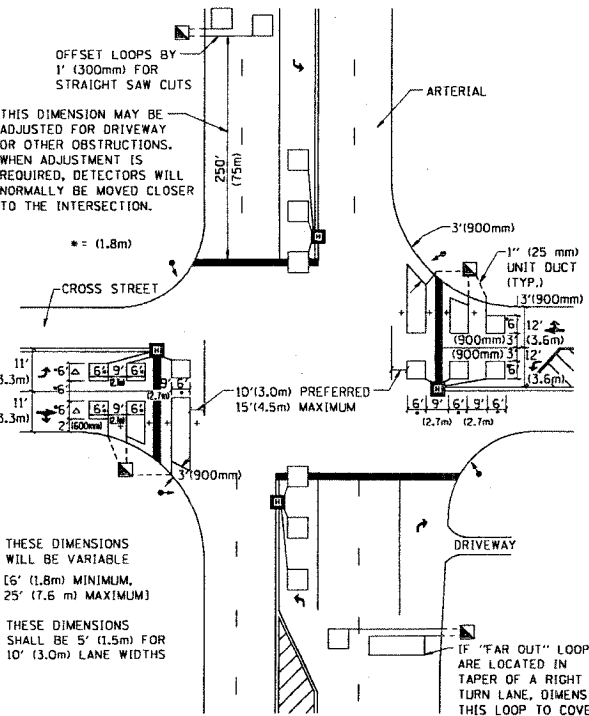
DETAIL 2 N.T.S.
