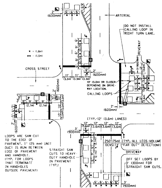
DETAIL 1 N.T.S.
