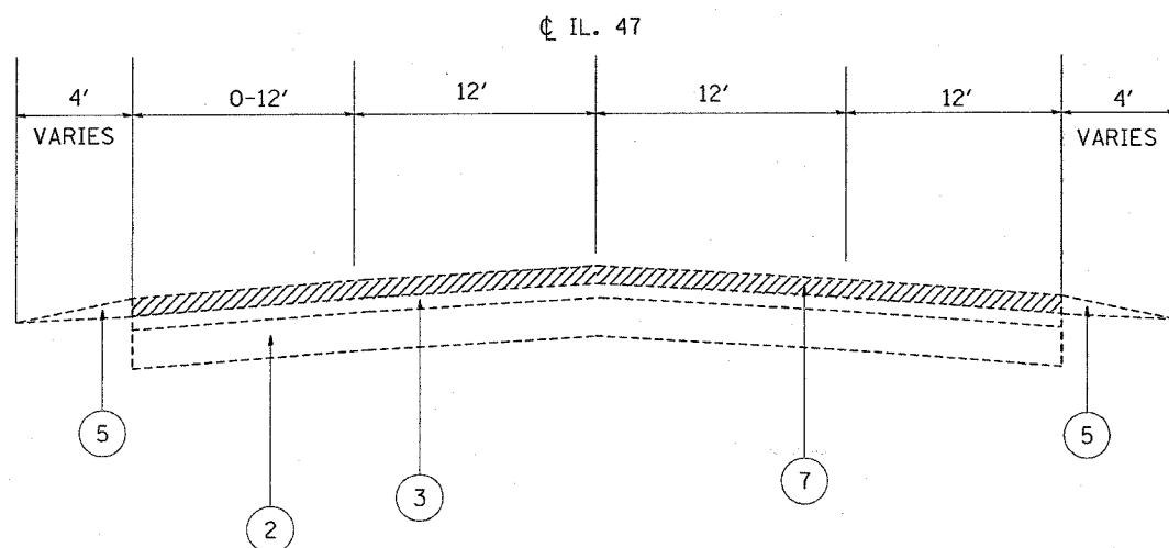
EXISTING TYPICAL SECTION STA. 24+00 TO STA. 32+00 STA. 73+00 TO STA. 90+00
