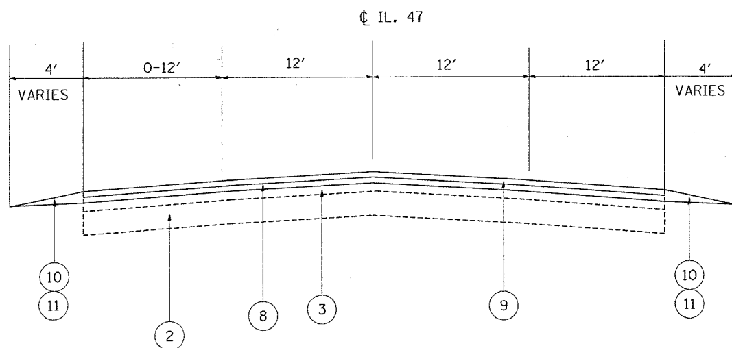
PROPOSED TYPICAL SECTION STA. 24+00 TO STA. 32+00 STA. 73+00 TO STA. 90+00
