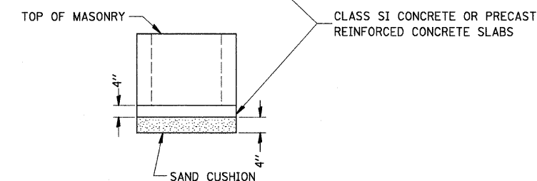
SEC. A-A
