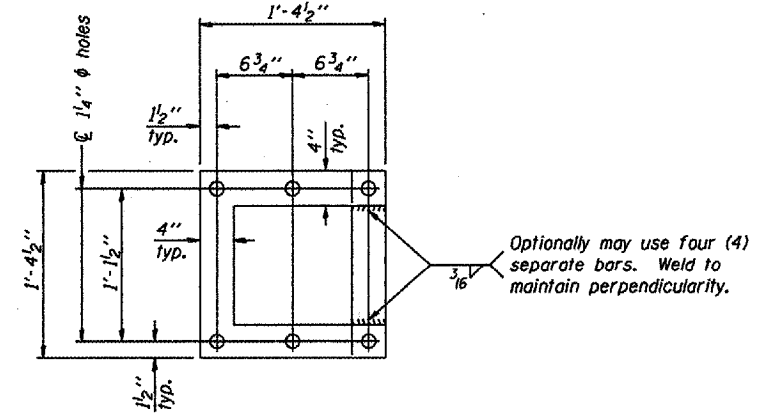
POSITIONING PLATE(S)
