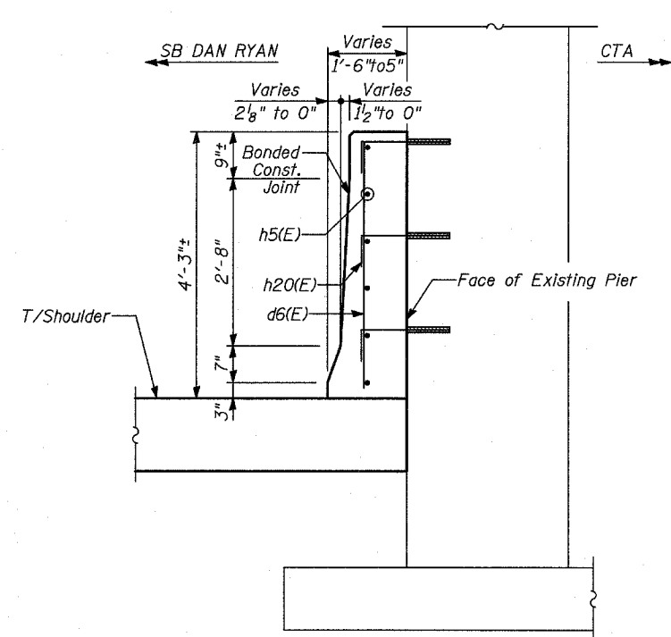
SECTION D-D
