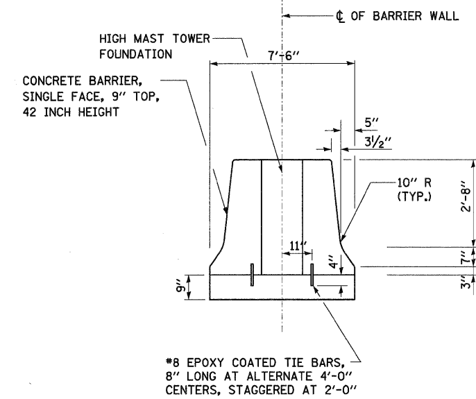
SECTION D-D
