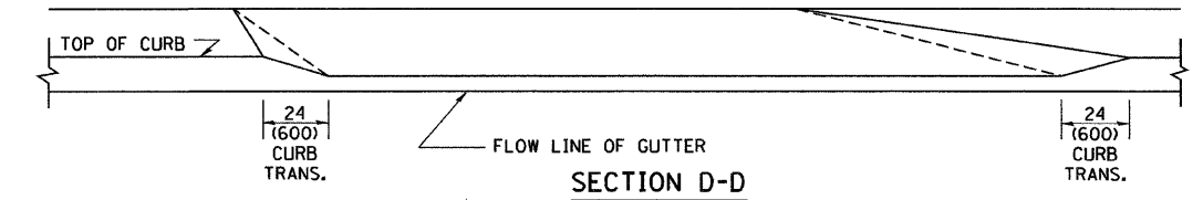
SECTION D-D
