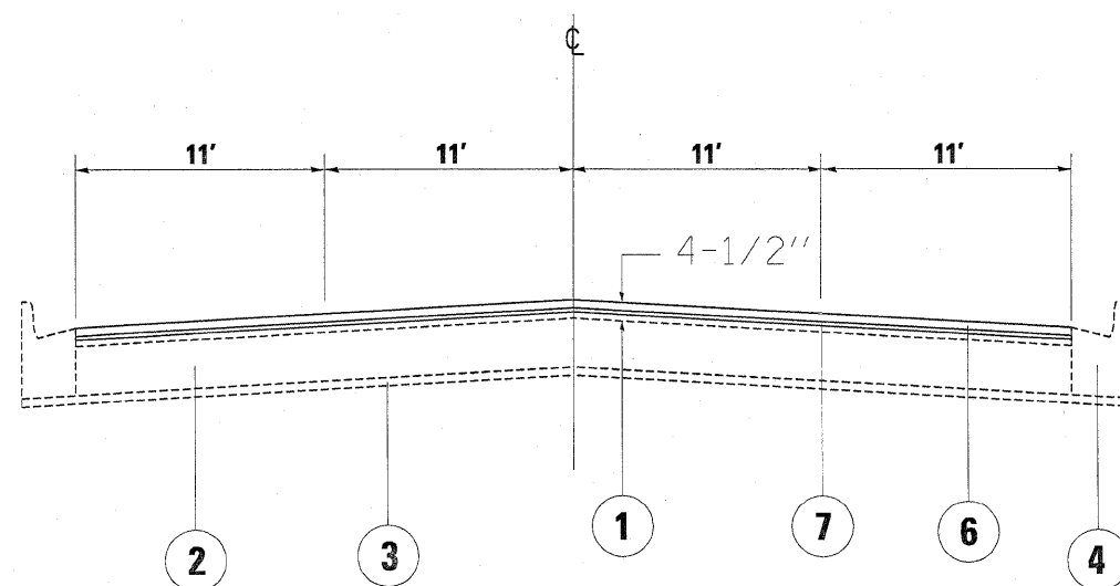
PROPOSED TYPICAL CROSS SECTION STA. 10+00 TO STA. 54+00 STA. 74+00 TO STA. 83+00
