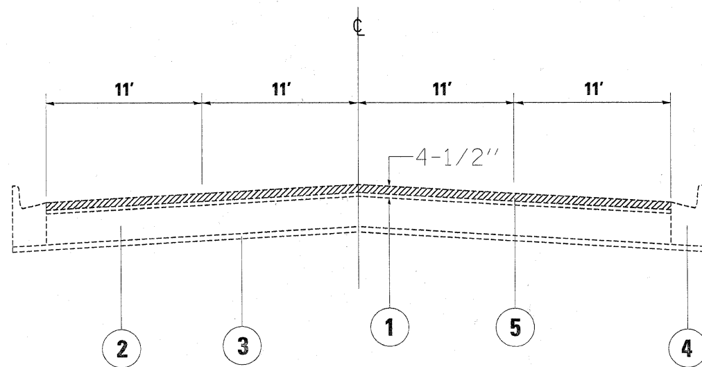
EXISTING TYPICAL CROSS SECTION STA. 10+00 TO STA. 54+00 STA. 74+00 TO STA. 83+00
