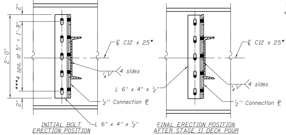
FINAL ERECTION POSITION AFTER STAGE II DECK POUR
