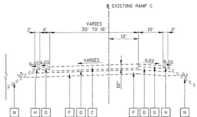
EXISTING TYPICAL SECTION RAMP C STA 7000+79 TO STA 7014+74
