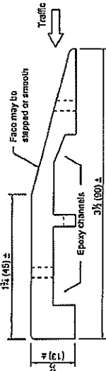
SECTION A-A
