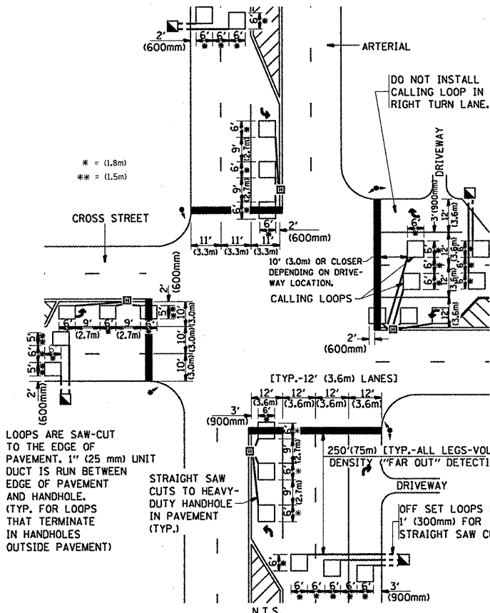
DETAIL 1 N.T.S.
