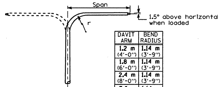
DAVIT ARM
