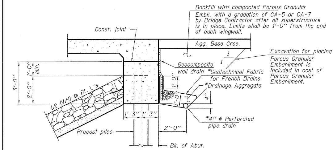
SECTION A-A (Horiz. dim. @ Rt. L's)
