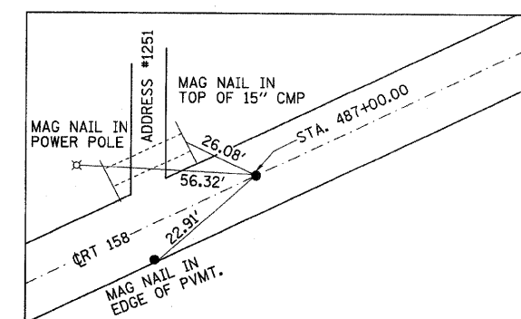
TIES TOP C POINT STA. 487+00.00 MAG NAIL N 656101.6547 E 2325321.4088
