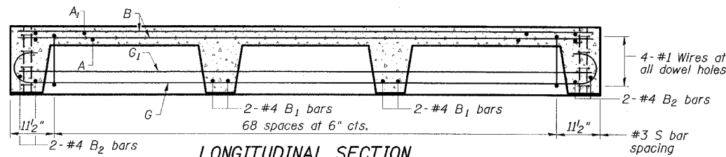
LONGITUDINAL SECTION
