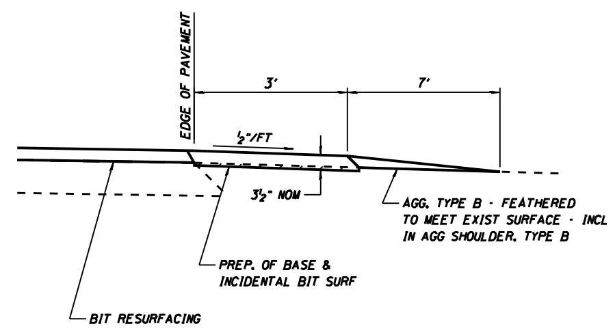
SECTION A-A FOR AGGREGATE PE
