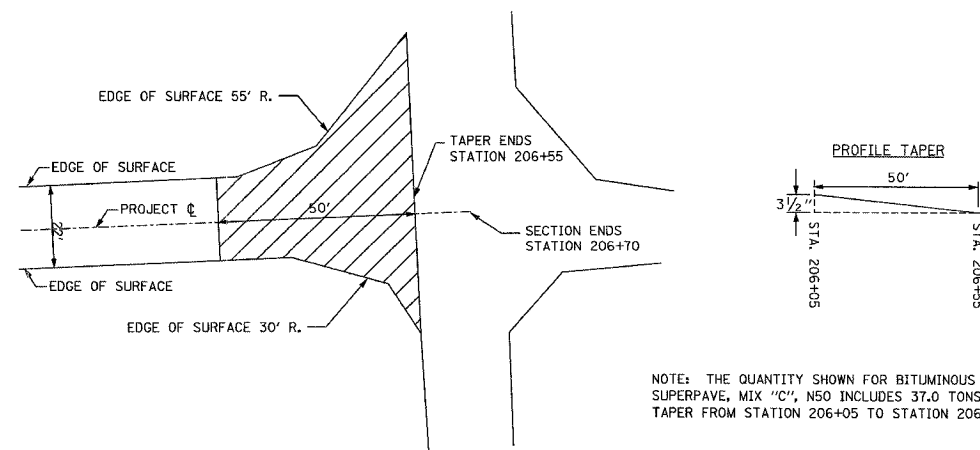
DETAIL OF TAPER STA. 206+00 TO STA 206+25
