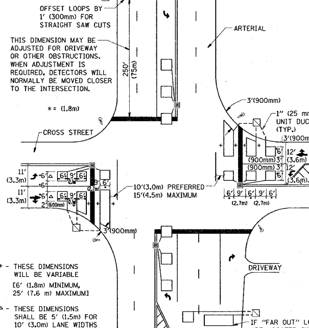
DETAIL 2 N.T.S.
