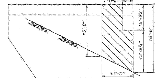
S. Abut. E. Wing - West Structure
