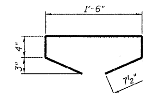
BAR G5
