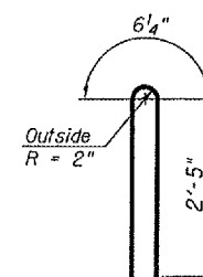
BAR G2
