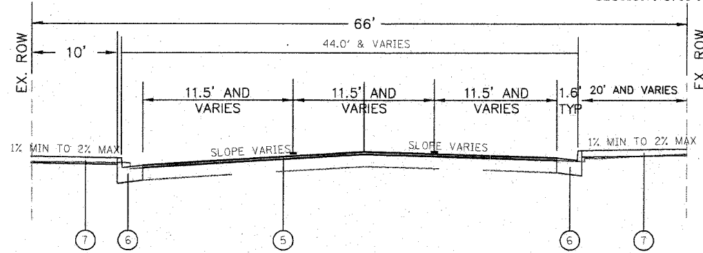
IL 159 (N. & S. ILLINOIS ST.) PROPOSED TYPICAL SECTION STA. 45+67.56 TO STA. 47+85.06 STA. 50+58.34 TO STA. 52+74.58
