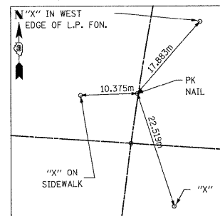
PI IL 47 - STA 20+945.776
