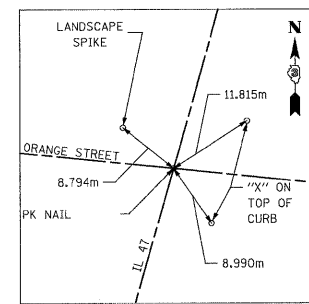
PC IL 47 - STA 20+351.279
