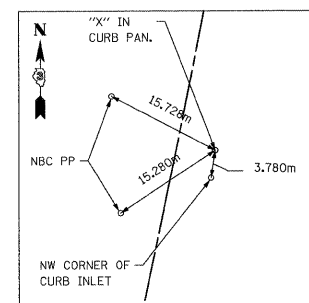
PI IL 47 - STA 20+507.892
