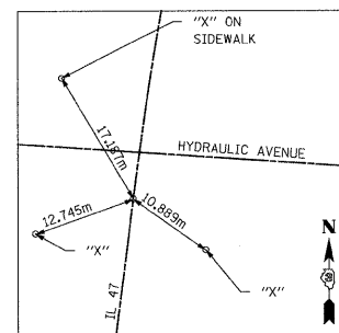
PC IL 47 - STA 20+930.534
