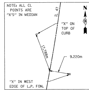
PRC IL 47 - STA 20+961.009
