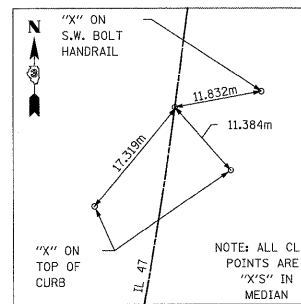
PT IL 47 - STA 20+991.460
