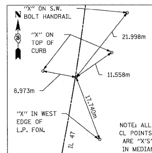
PC IL 47 - STA 20+976.238
