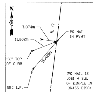
PT IL 47 - STA 20+663.918
