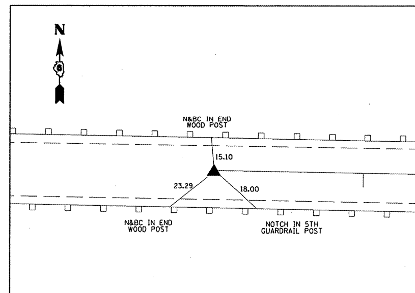
STA 591+76.62
