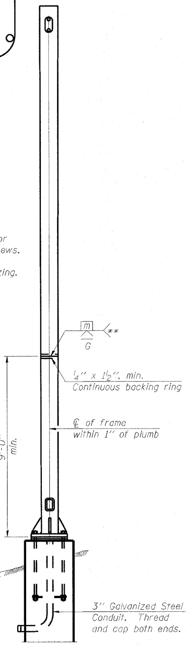
END ELEVATION
