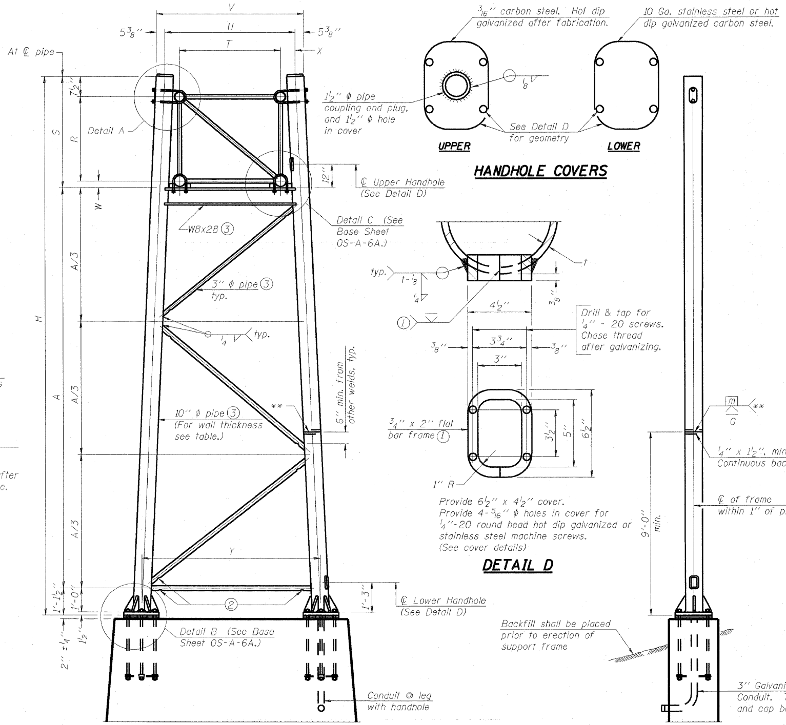
END ELEVATION
