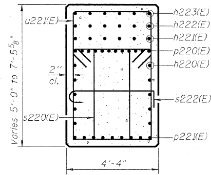
SEC. A-A
