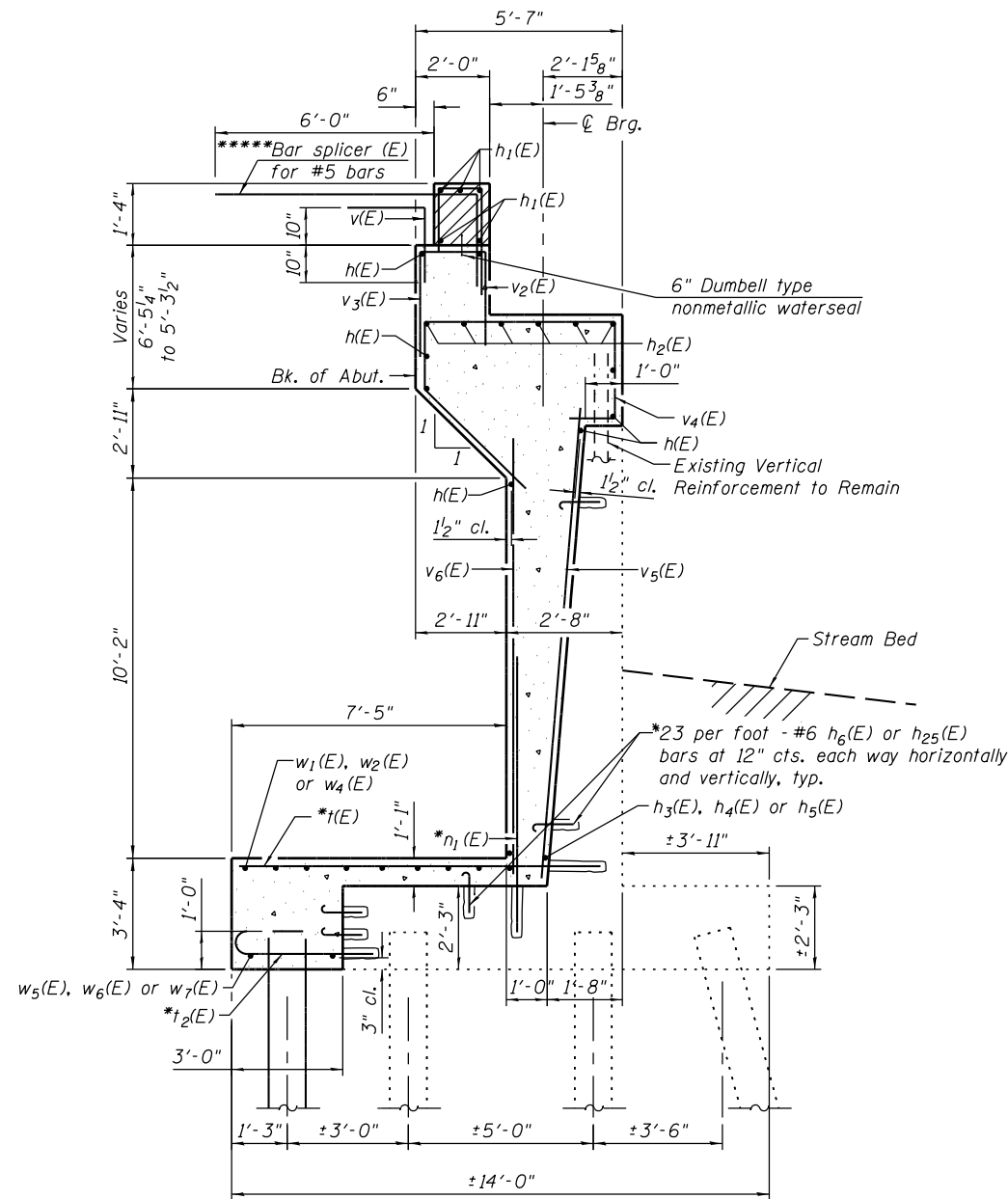
SECTION A-A
