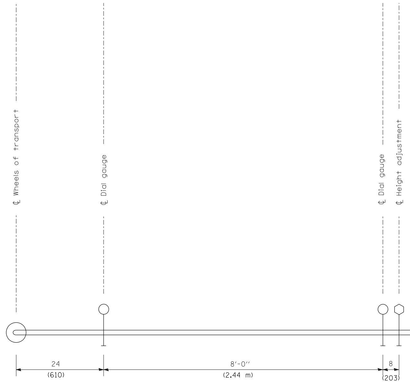
ELEVATION
