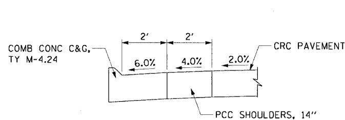
SECTION C-C N.T.S.
