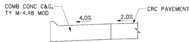
SECTION A-A N.T.S.
