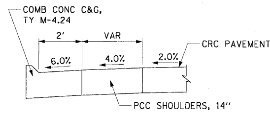
SECTION D-D N.T.S.
