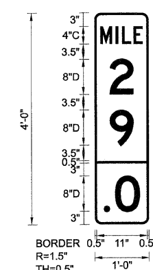
EB-MM-59 STA. 1170+60
