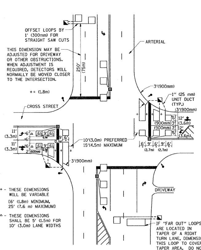
DETAIL 2 N.T.S.
