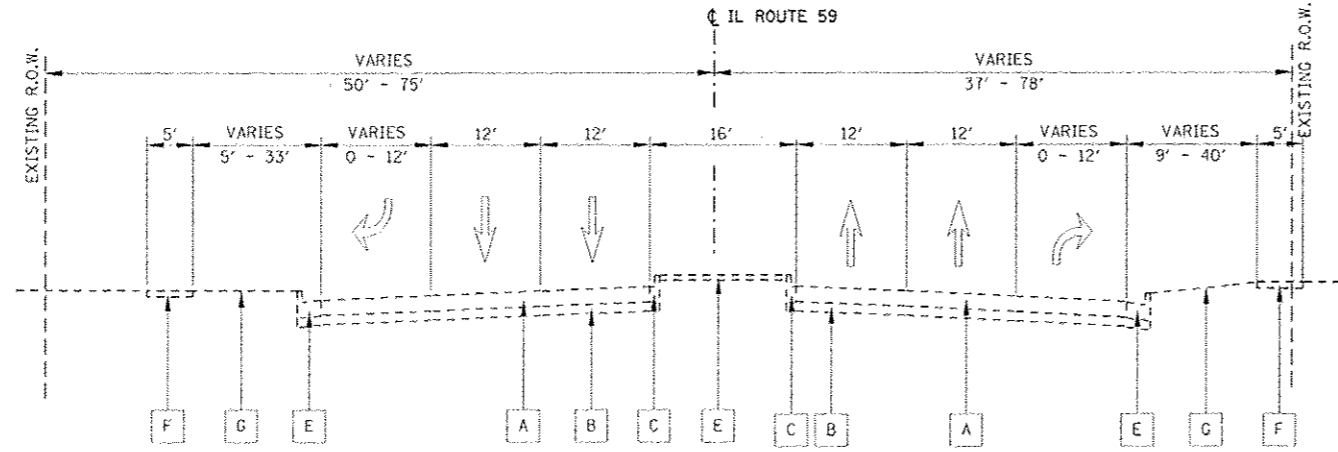
FULL WIDTH MEDIAN STA. 3988+84 TO STA. 3989+65 STA. 4006+41 TO STA. 4009+88 STA. 3994+17 TO STA. 4002+03 STA. 4020+03 TO STA. 4027+23
