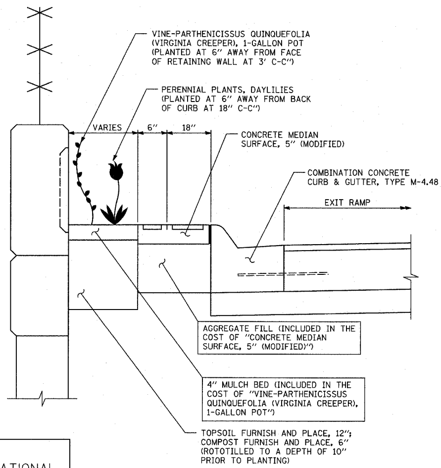
SECTION A-A
