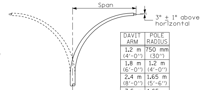
DAVIT ARM
